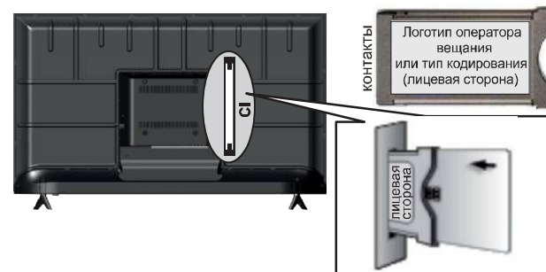
Рисунок 5 – Установка СА-модуля
