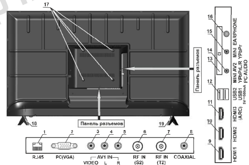
1 – вход RJ45 для подключения к сети Интернет; 2 – вход PC(VGA) для подключения видеосигнала с компьютера; 3 – вход видео VIDEO композитного разъема AV1 IN ; 4 – вход звука L композит-
