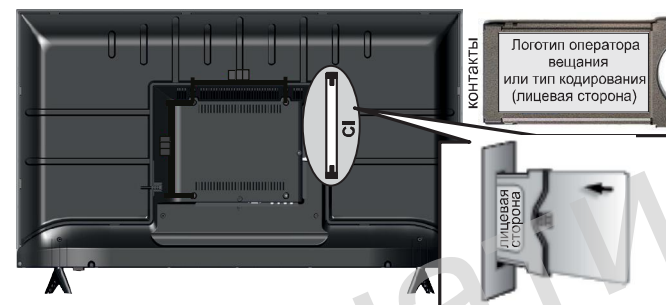
Рисунок 4 – Установка СА-модуля
