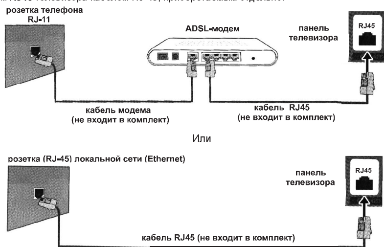
Рисунок 5 – Проводное подключение
