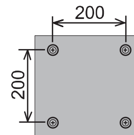
Рисунок 3 – Размеры для выбора настенного кронштейна
