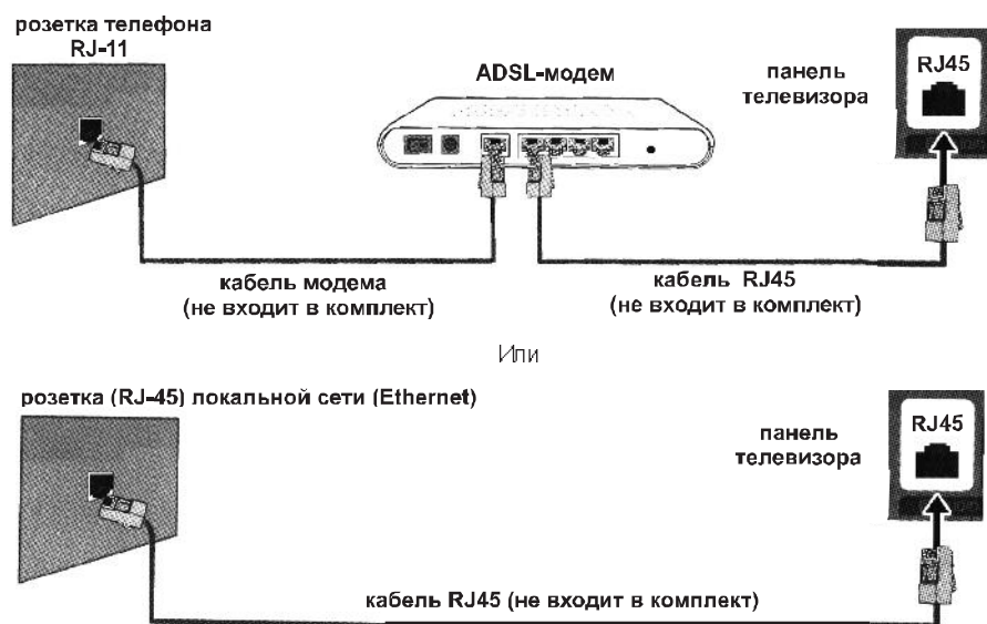
Рисунок 5 – Проводное подключение
