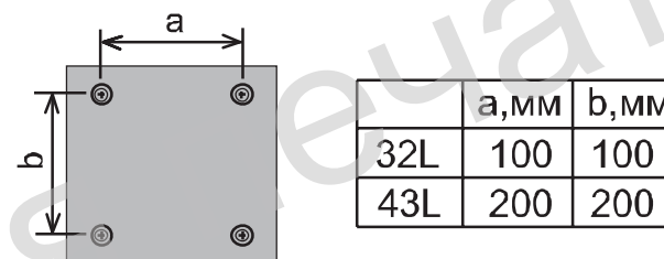
Рисунок 3 – Размеры для выбора настенного кронштейна
