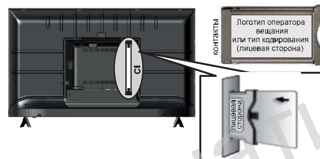
Рисунок 4 – Установка CA-модуля
