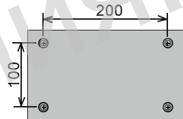
Рисунок 4 – Размеры для выбора настенного кронштейна
