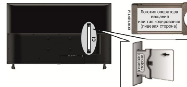
Рисунок 5 – Установка СА-модуля
