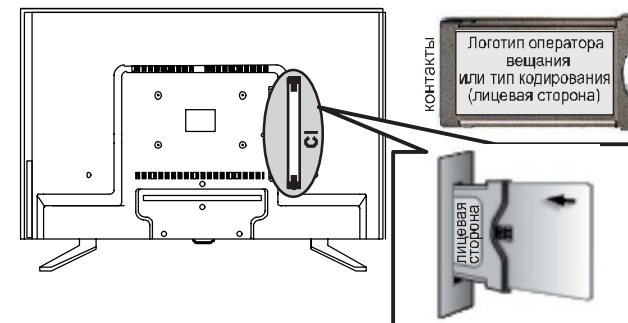
Рисунок 7 – Установка CA-модуля
